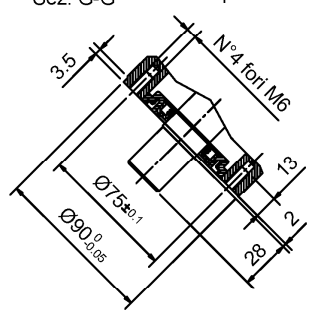
Sez. G-G
